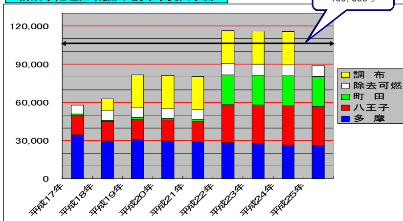
構成市処理区域拡大・調布市受入予測
